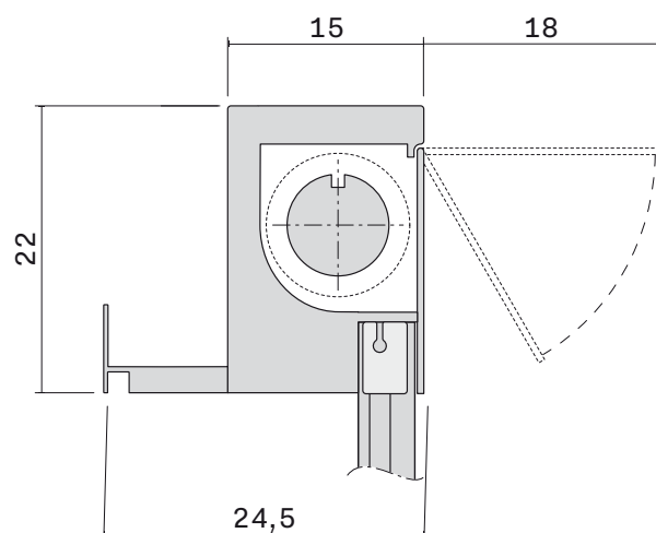
TARTÓGERENDA 15 X 22
