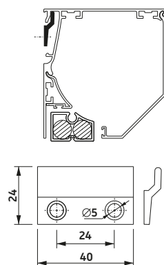
TOK TARTÓ
