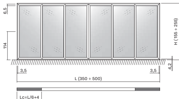
3 SÍN - 6 AJTÓ
