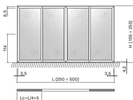
2 SÍN - 4 AJTÓ
