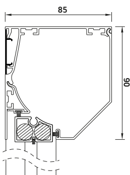
ZÁRÓLÉC
