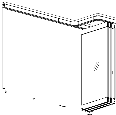
HARMONIKAÜVEG D-10
