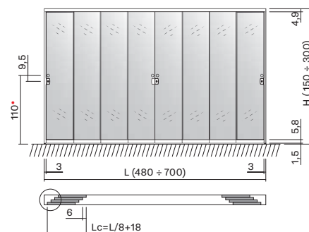
4 SÍN - 8 AJTÓ
