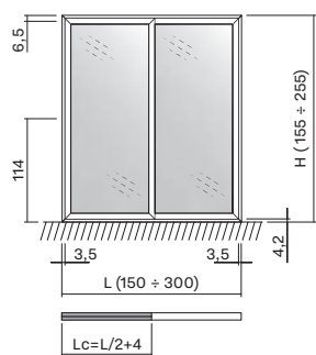
2 SÍN - 2 AJTÓ
