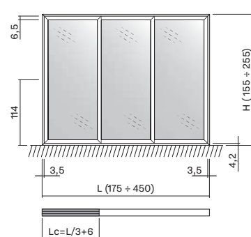
3 SÍN - 3 AJTÓ
